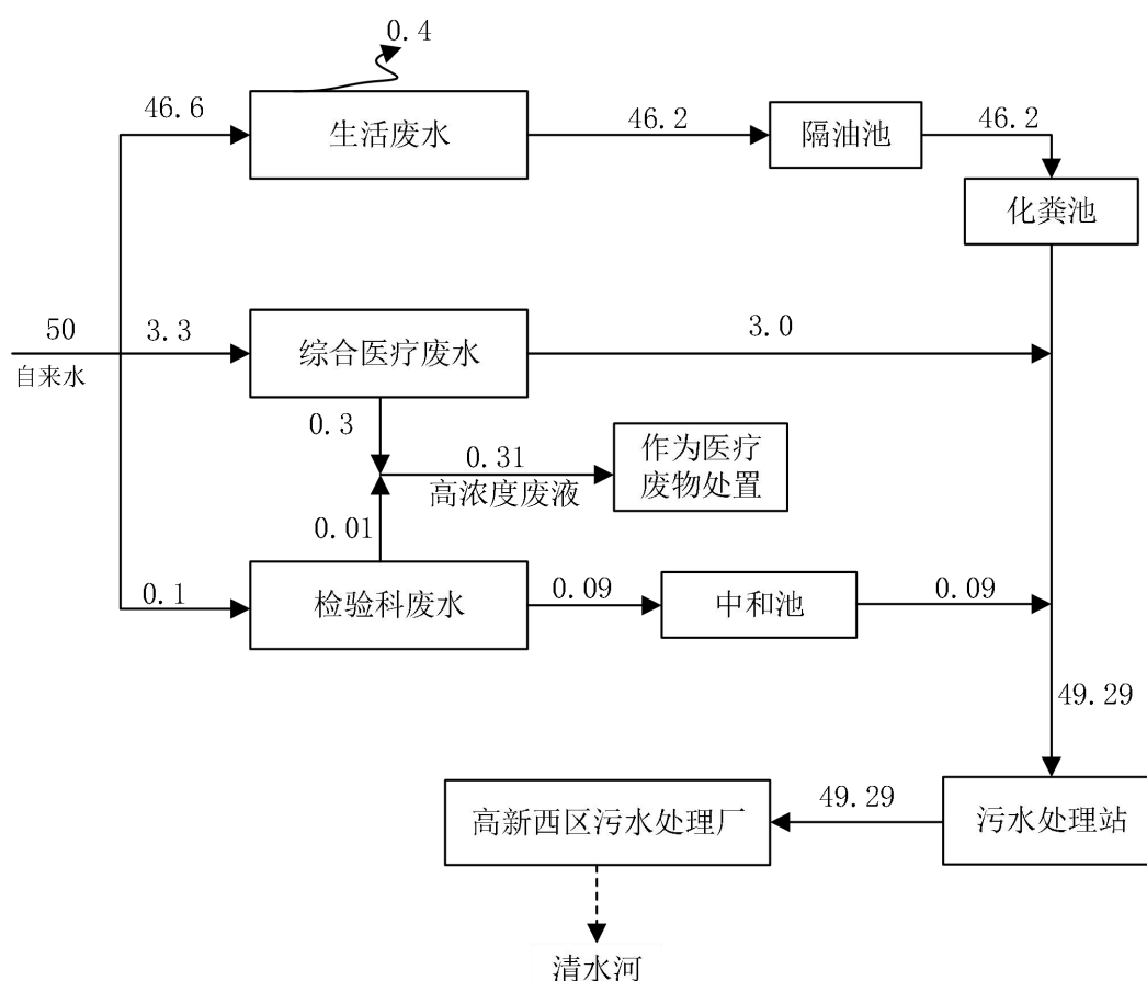
图 3-1 项目水平衡图 ( \text{m}^3/\text{d} )
